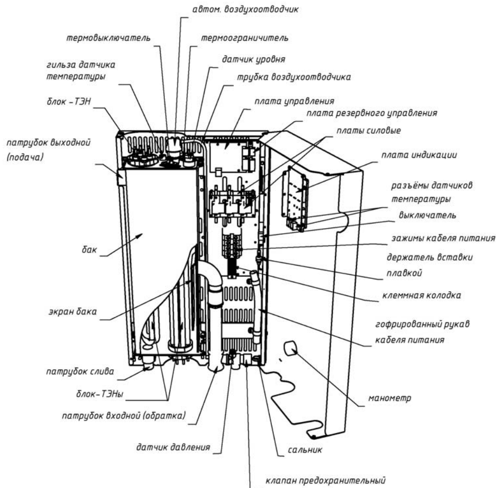
Рис. 4. Устройство прибора
